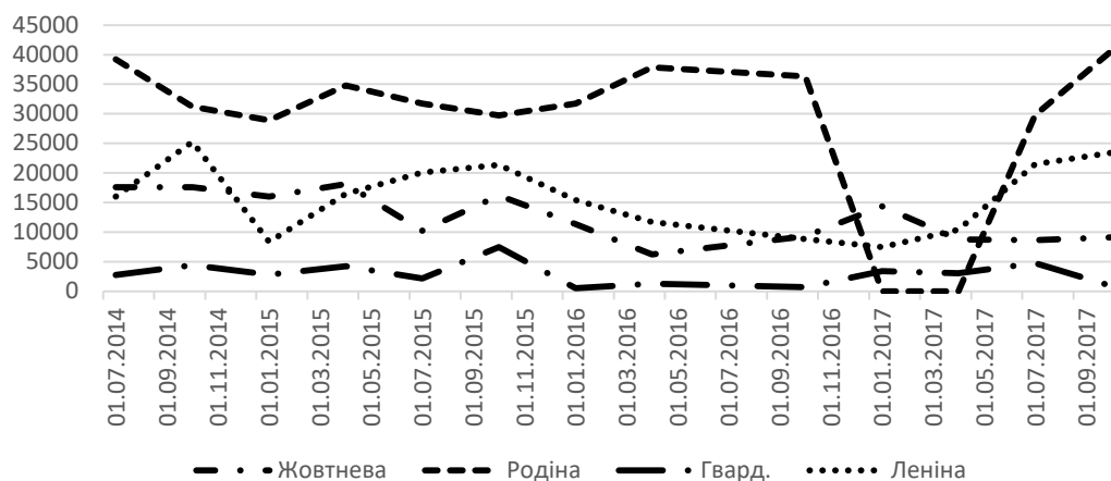
Рис. 2. Споживання електроенергії на водовідливних установках залізрудних шахт Кривбасу
