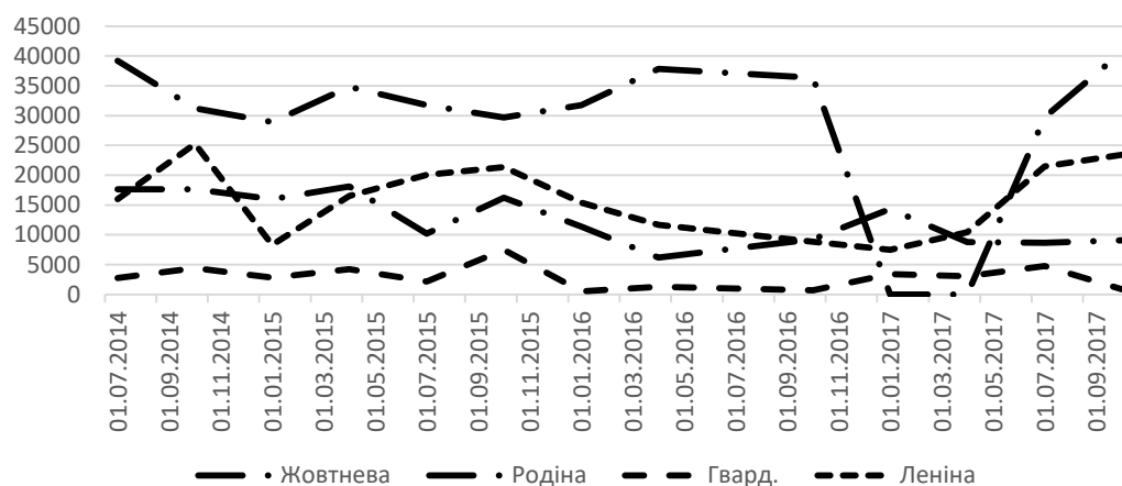
Рис. 3. Споживання електроенергії на вентиляційних установках залізрудних шахт Кривбасу
